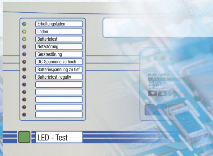
3 LED-Meldekarte
