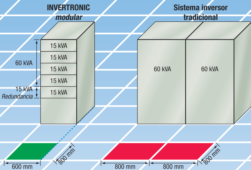
Fig. 6: Comparación de sistemas inversores redundantes n+1
